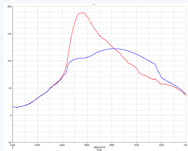
Figura 18 – Idrogrammi T100 anni in corrispondenza dell'area di laminazione di Chiodello (Scenario 4)
